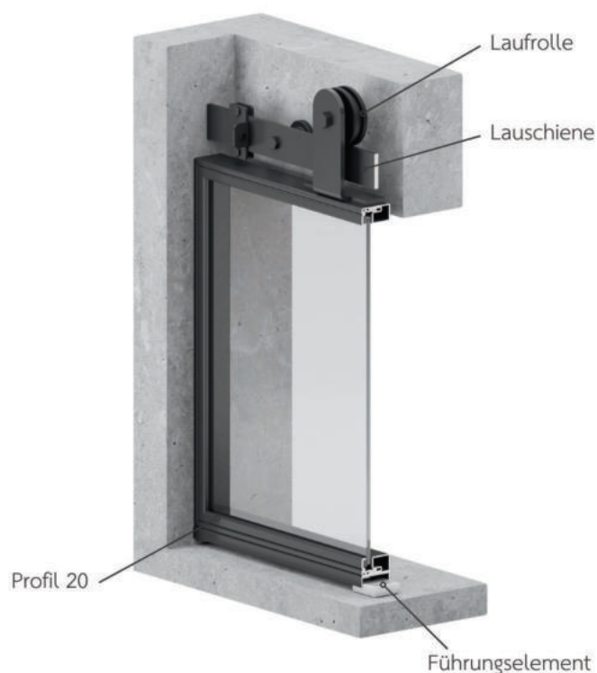
Ansicht bei Wandmontage
